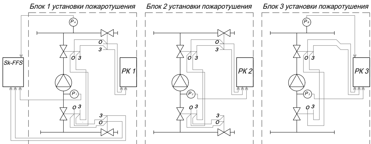
Рис. 1. Схема блоков
